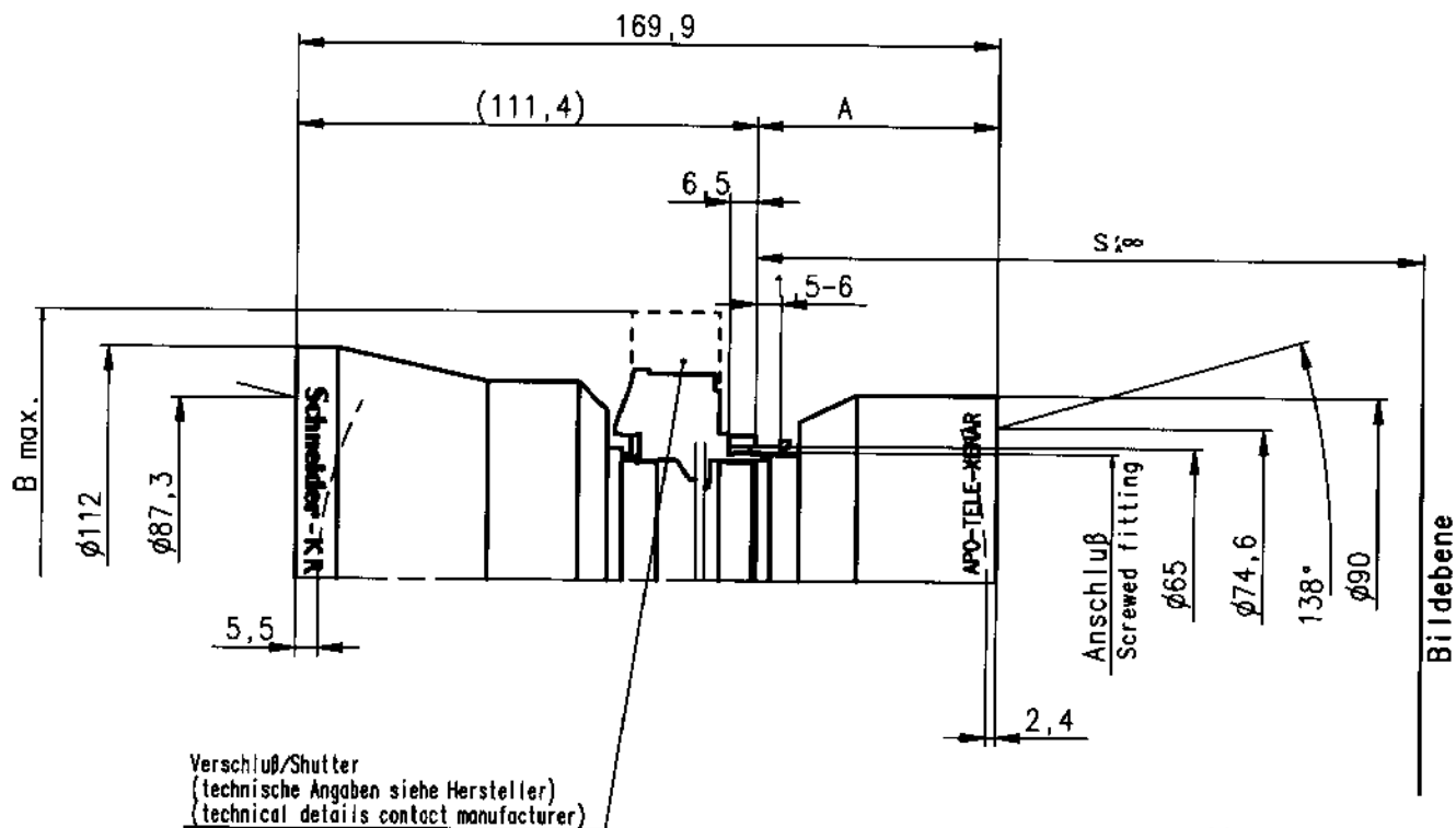
APO-TELE-XENAR 12,0/800 in Verschluß 3 Shutter 3
